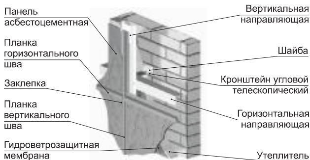
Рис. 1. Основные элементы конструкции системы МК1-02
