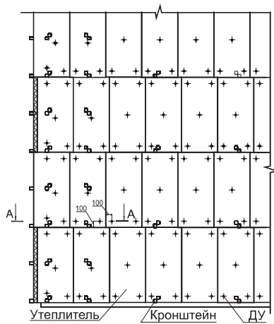
Рис. 4. Принципиальная схема установки 1-го слоя при однослойном и 2-го слоя при двухслойном утеплении
