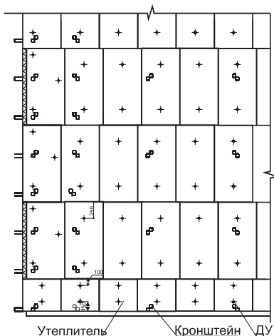
Рис. 3. Принципиальная схема установки 1-го слоя при двухслойном утеплении
